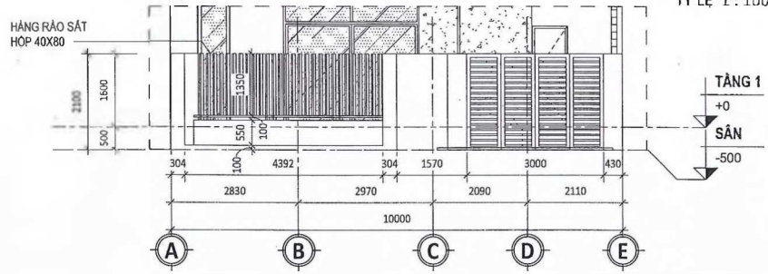
MẶT ĐỨNG A-E ( CỔNG HÀNG RÀO ) TỶ LỆ 1:100
