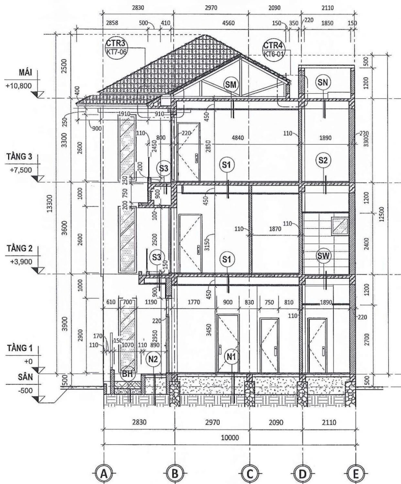
MẶT CẮT 3-3 TỶ LỆ 1 : 100
