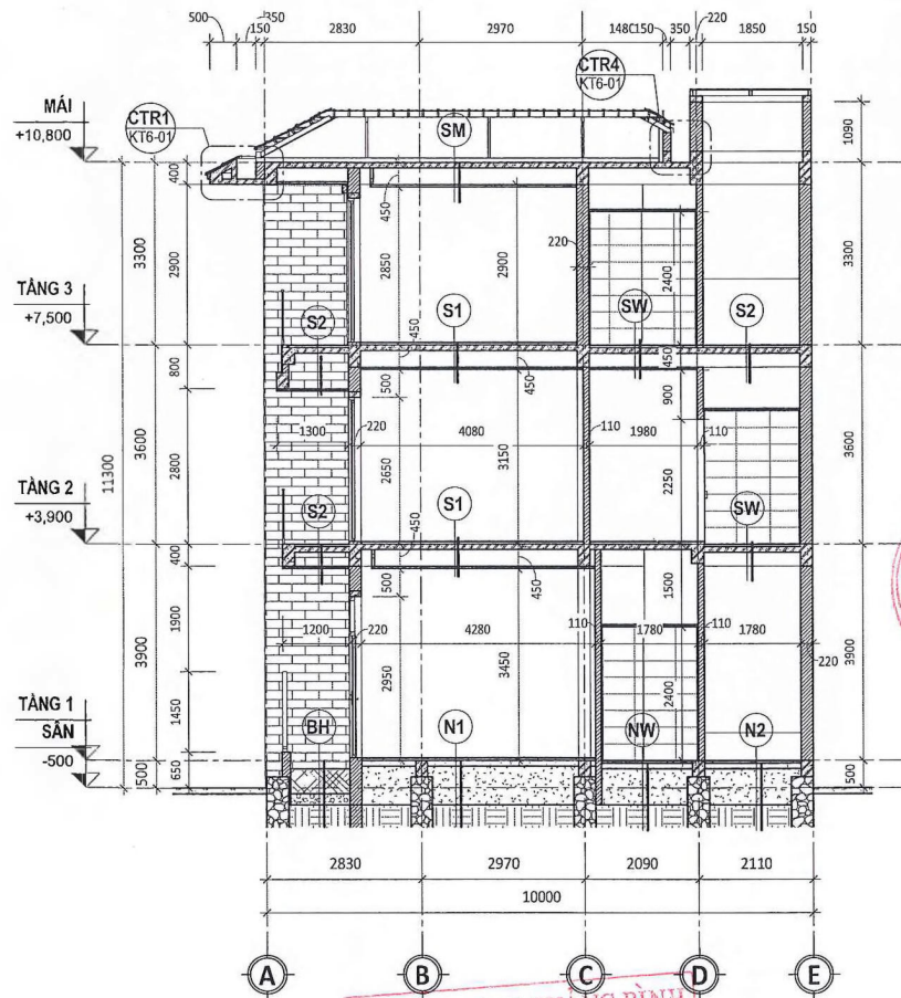
MẶT CẮT 4-4 TỶ LỆ 1 : 100
