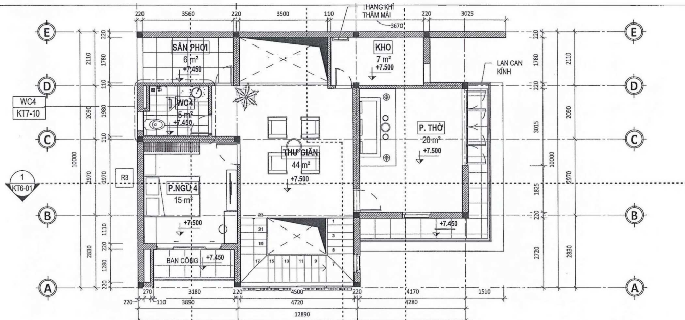
MẶT BẰNG TẦNG 3
